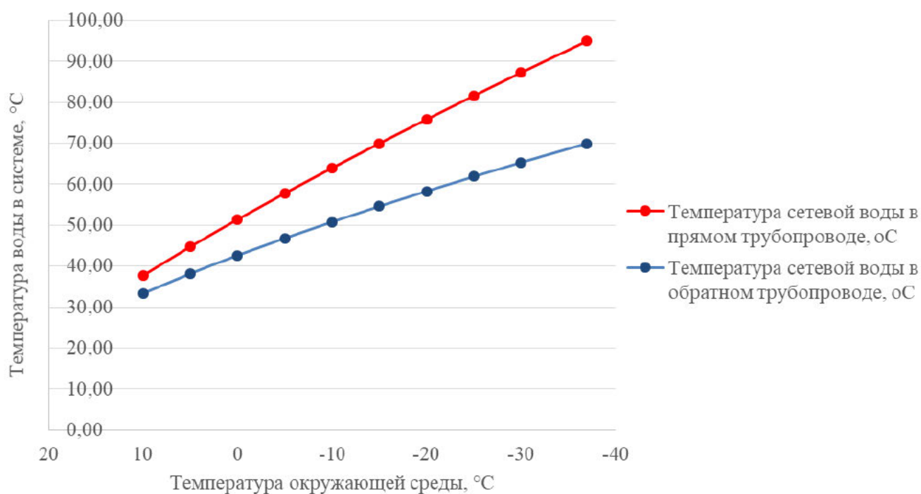
Рисунок 2.2 – График изменения температур теплоносителя (температурный график 95/70^{\circ}\text{C} )
