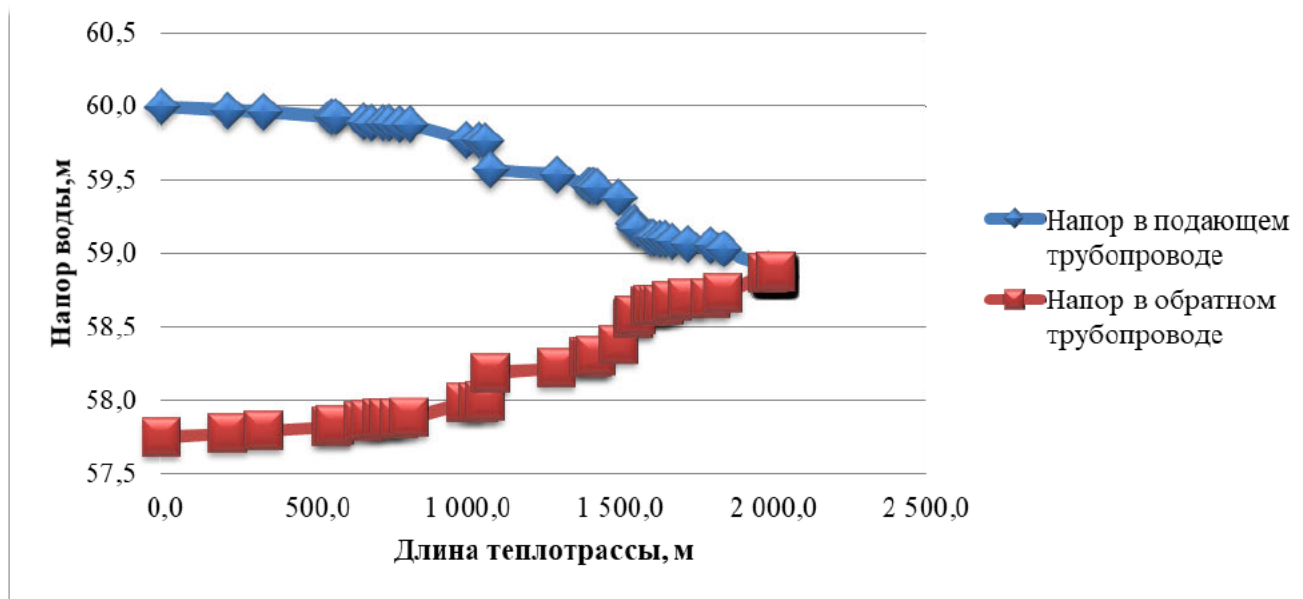
Рисунок 2.3 – Пьезометрический график тепловой сети котельной «Новый Урал» по магистральному выводу
